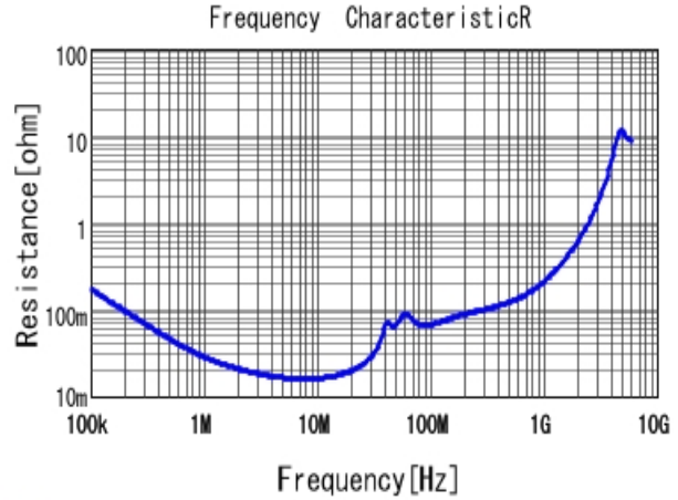
■ GRM21BR71E104KA01 R DCOV, 25degC
