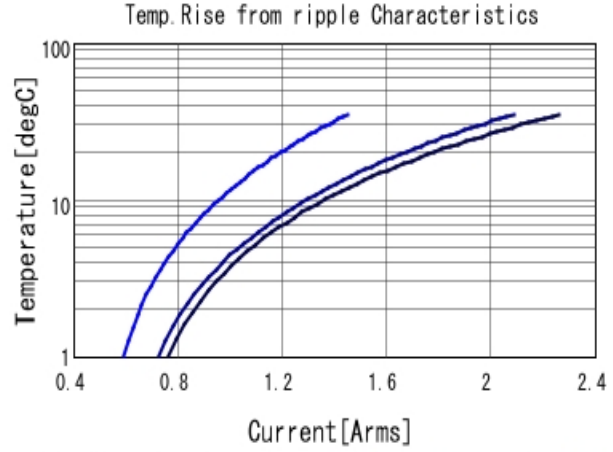
GRM21BR71E104KA01 Temp. rise ■ 400kHz ■ 800kHz ■ 1MHz
