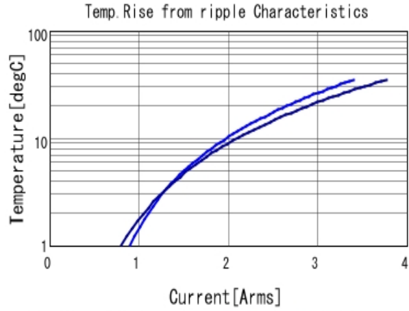
GRM219R71E105KA88 Temp. rise ■ 500kHz ■ 1MHz
